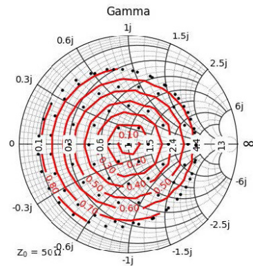
96 GHz, \Gamma_{max} : 0.839
