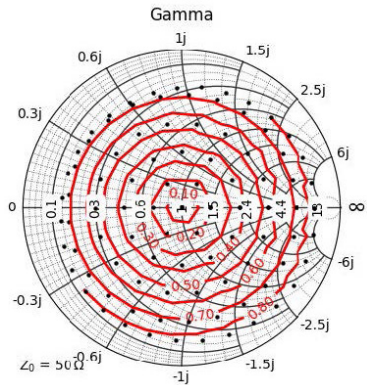
28 GHz, \Gamma_{max} : 0.839
