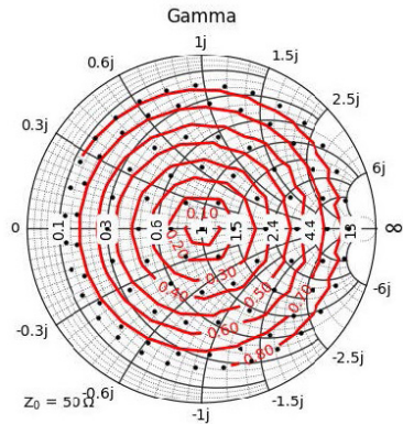
50 GHz, \Gamma_{max} : 0.844
